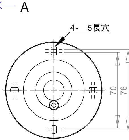
取付け仕様 (A矢視図)
