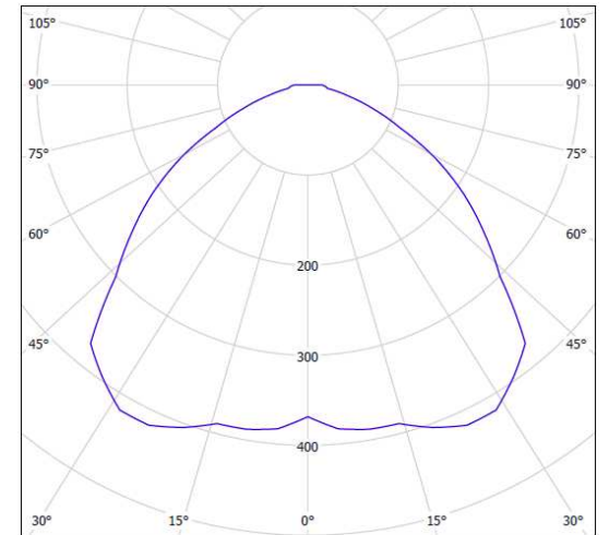
【配光図】 1/2ビーム角 : 110°
