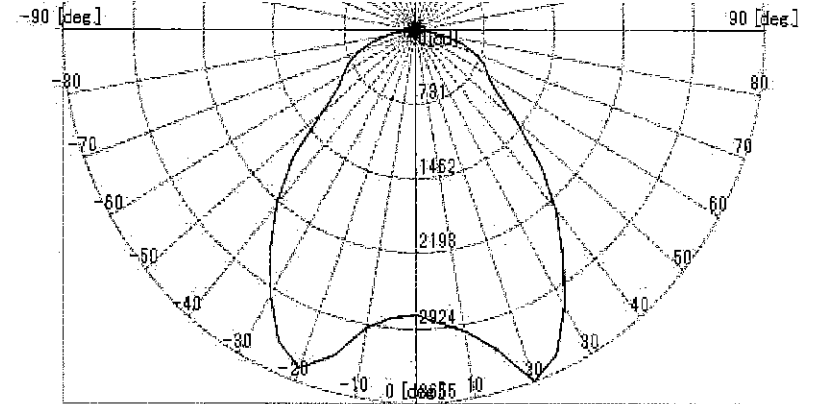
【配光図】 PL-480A-C120W
