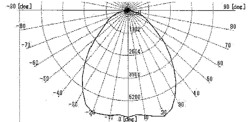
【配光図】 PL-564A-CC200W, PL-564A-CC260W
