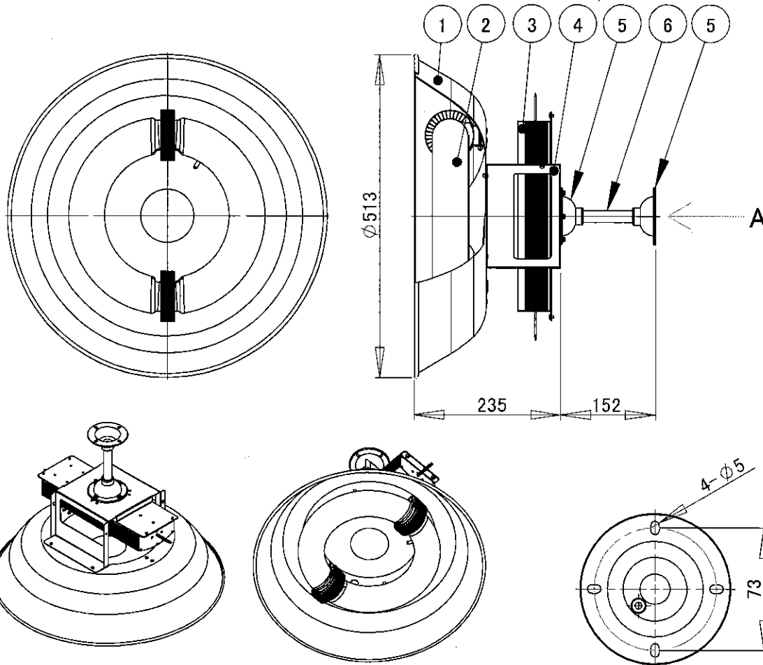
取付け仕様(A矢視図)
