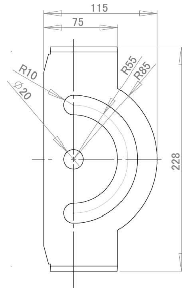
取付け仕様 (A矢視図)
