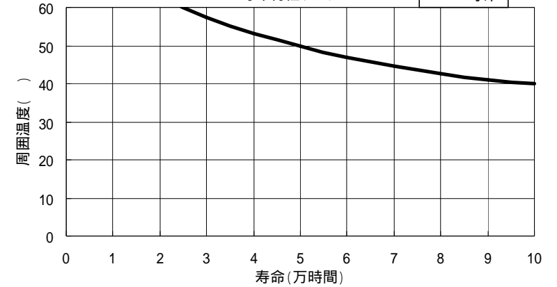
寿命特性グラフ
