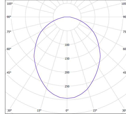
【配光図】 1/2ビーム角: 100° [cd/klm]
