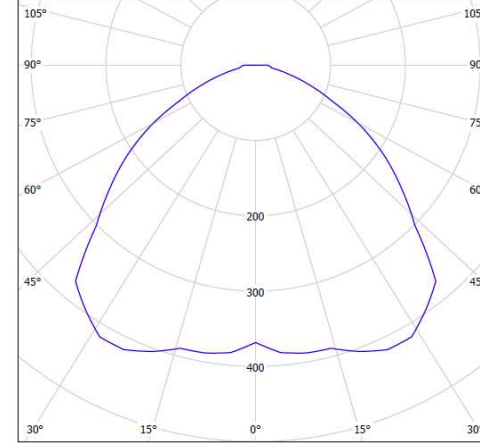
【配光図】 1/2ビーム角 : 110° (cd/klm)
