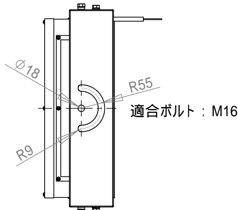
【取付け部寸法】
